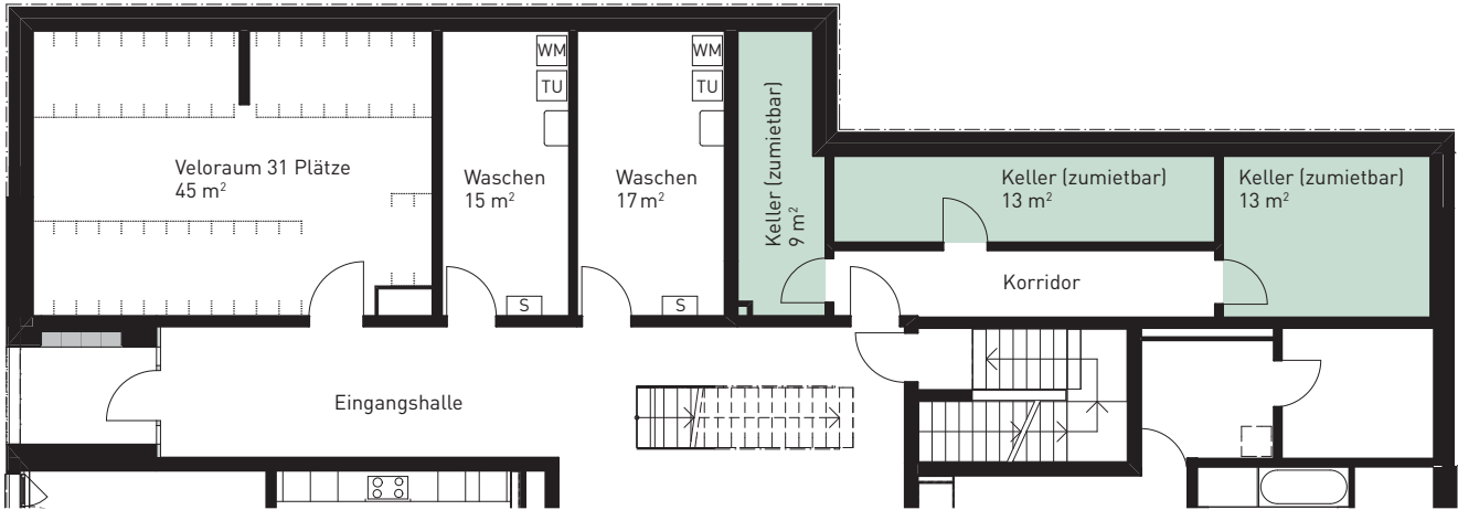
ERDGESCHOSS
