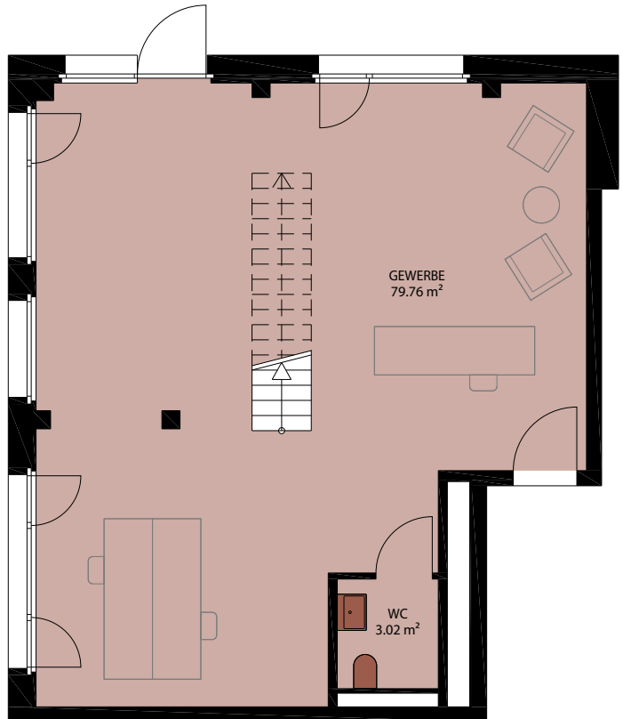
ERDGESCHOSS
